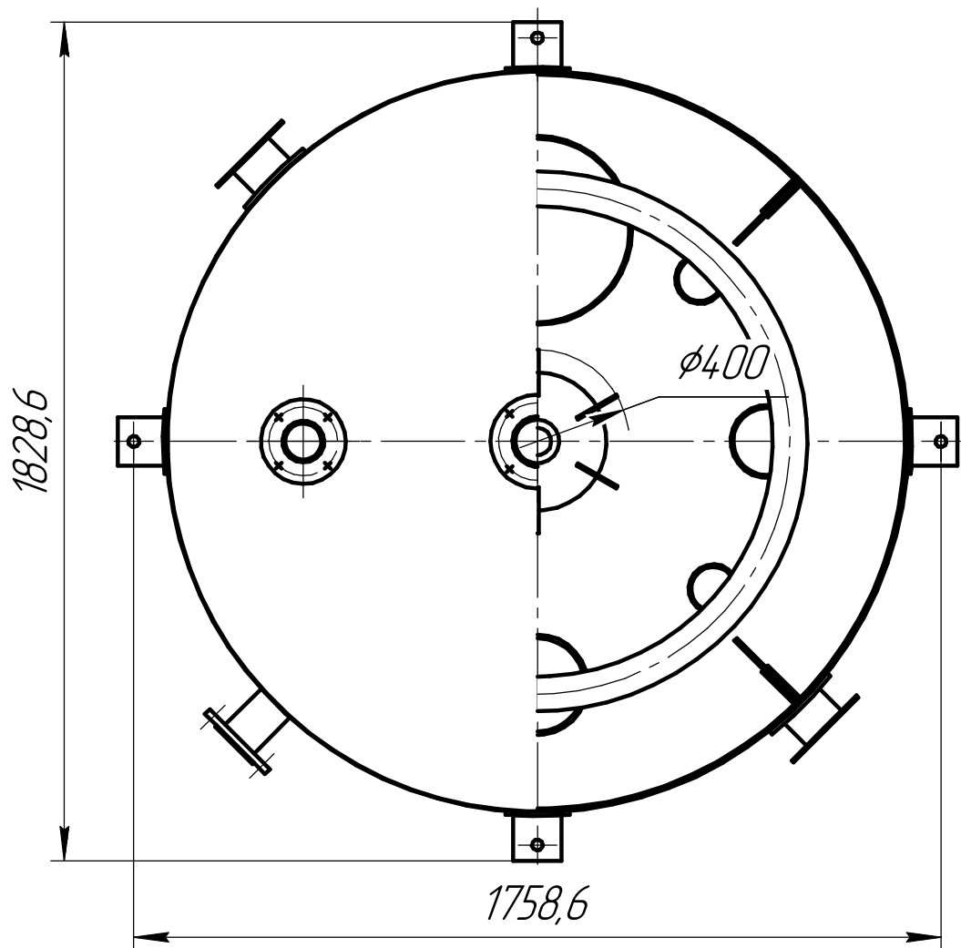
Б(1:15)
