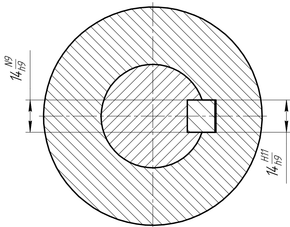
Д-Д(1:1)
