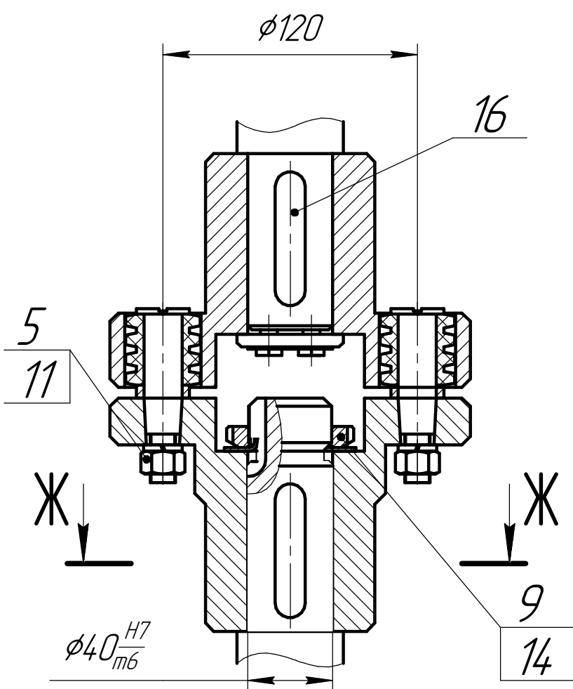
Е-Е(1:2,5)
