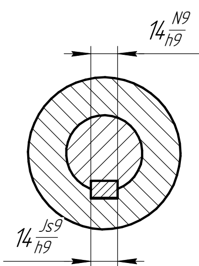
Ж-Ж(1:2)
